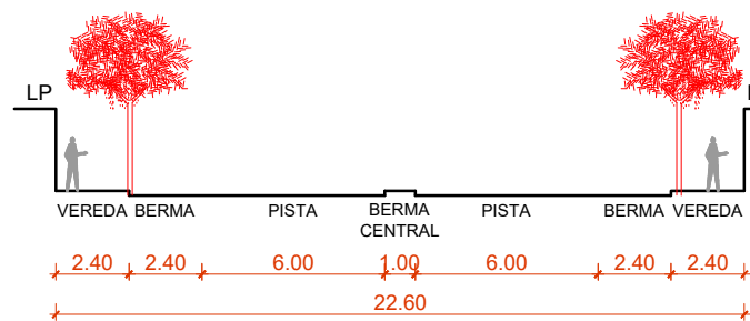
SECCION C-C: CALLE 1 VÍA DE INTERCONEXIÓN SANTA ROSA - ANCÓN
