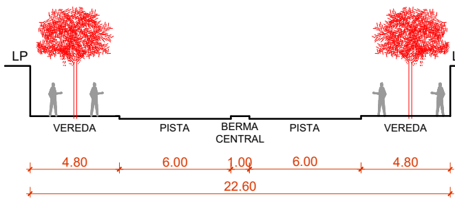
SECCION B-B: CALLE 1 VÍA DE INTERCONEXIÓN SANTA ROSA - ANCÓN
